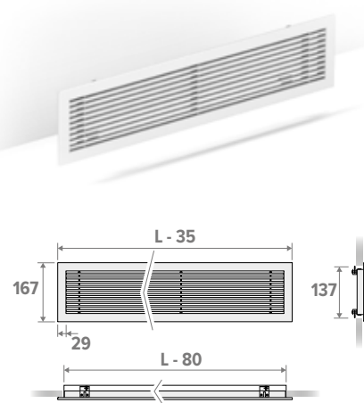
GRILLE À BARREAUX POUR PIÈCE D'ANGLE À 90°
