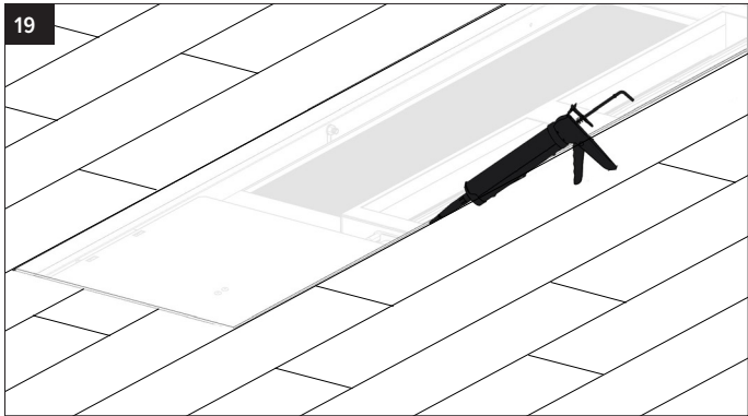
Werk rondom af.
