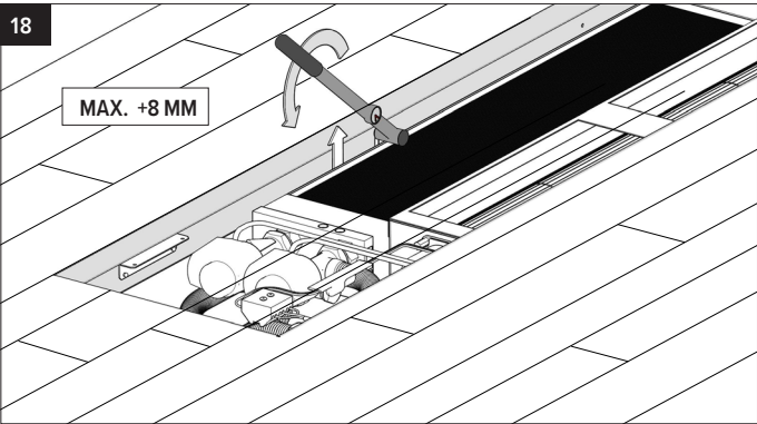
Fijnafstelling tot max. 0,8 cm voor een perfecte uitlijning met de afgewerkte vloer.
