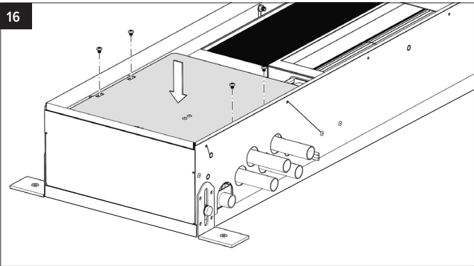
Monteer de ventiel afdekplaat.
