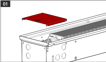
Démontez le couvercle de la vanne avant d'installer l'appareil
