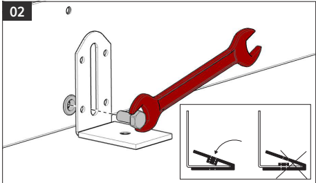
Plaats de hoogteregelingen aan de behuizing. Draai de bout niet volledig vast.
